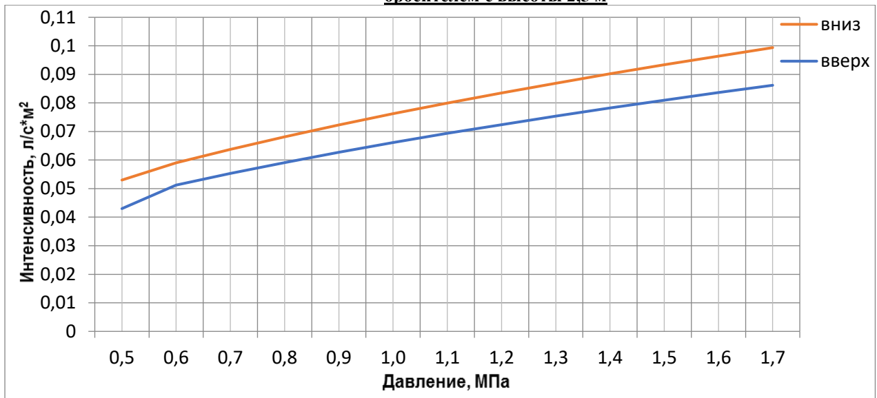
График зависимости интенсивности орошения от давления на площади 9 м 2 , защищаемой группой оросителей (два и более) с высоты 2,5 м
