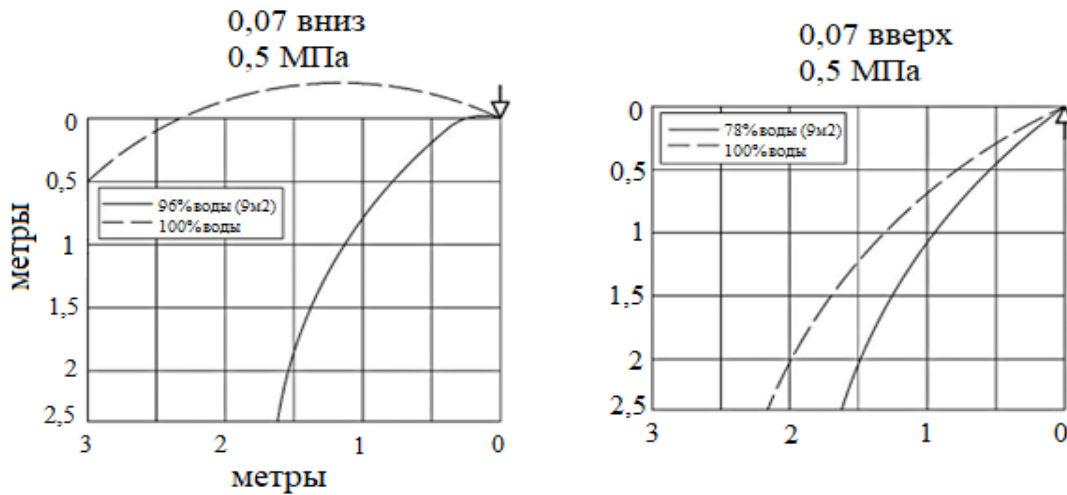
График зависимости интенсивности орошения от давления на площади 9 м 2 , защищаемой одним оросителем с высоты 2,5 м
